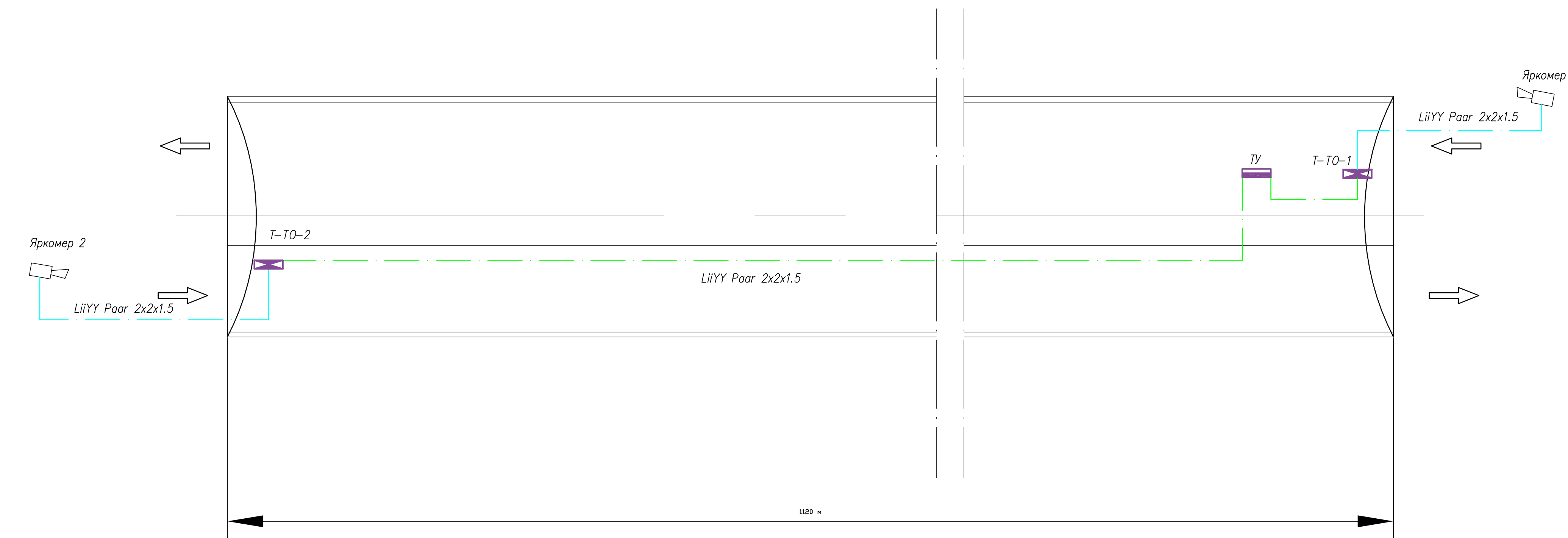
Схема на управление на тунелните осветителни уредби /ТОУ/
